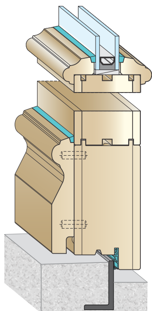
OPCIJA PROFILIRANO (zastekl. letvica, odkapna letev) AV-02 pohodni prag
