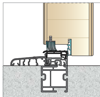
OPCIJA HH 80 BKV 80 TB pohodni prag
