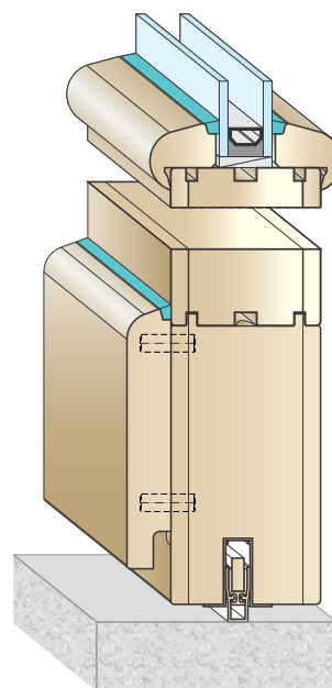
OPCIJA ZAobljeno (zastekl. letvica, odkapna letev) AV-07 pohodni prag
