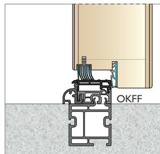
STANDARDNO HH 80 BKV 40 TB pohodni prag
