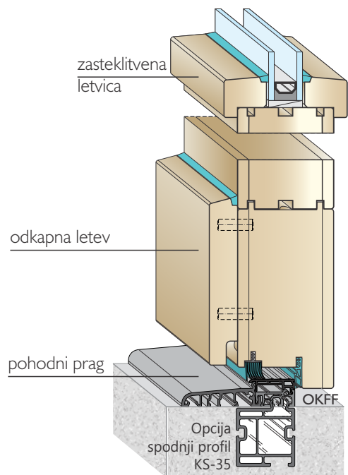
STANDARDNO HH 68 OGLATO (zastk. letvica in odkapna letev) BKV 80 TB pohodni prag
