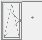
Balkonska vrata s fiksno zasteklitvijo (11-08 HA80-V)
