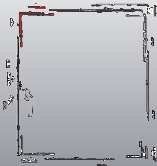
MVS-Kontaktelement
