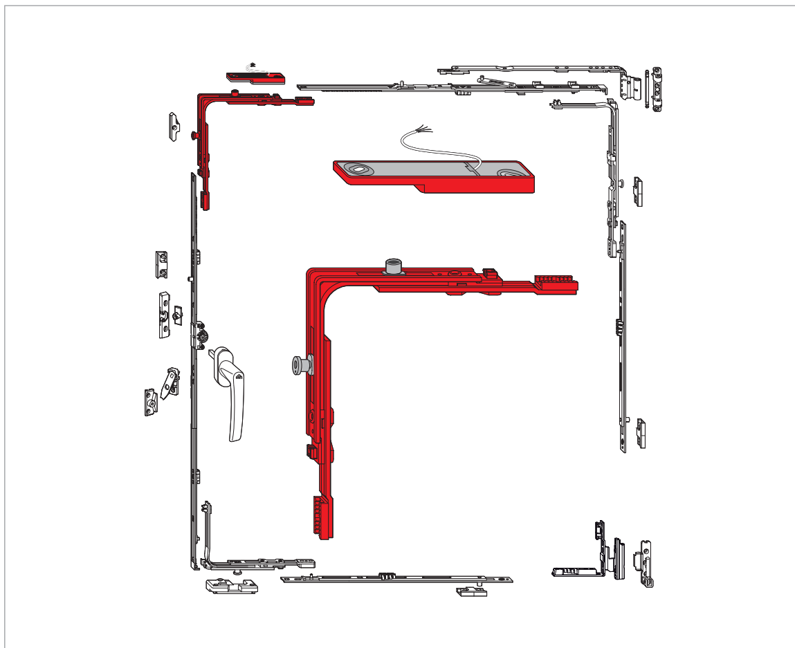
I-krilno okno
